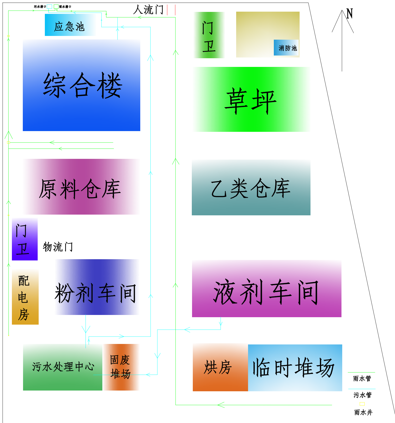
附图5 雨污分流图
